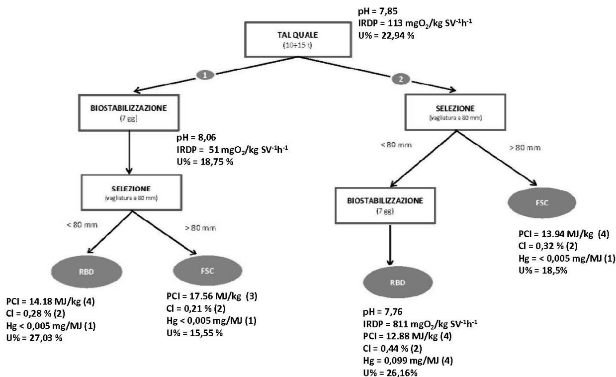
Figura 14. Schema dei trattamenti della sperimentazione e principali risultati ottenuti
