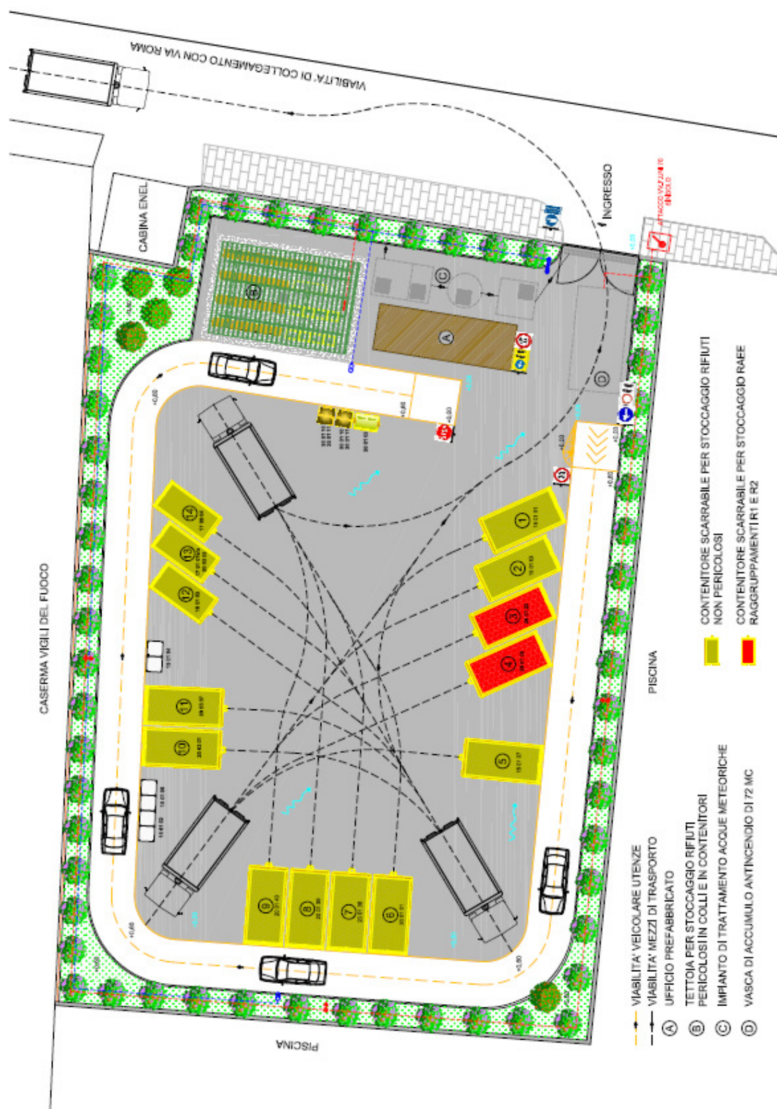
Figura 2 – Planimetria tipo di Centro Comunale di Raccolta
