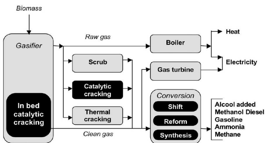
Fig. 13: processi catalitici applicabili alla gassificazione
