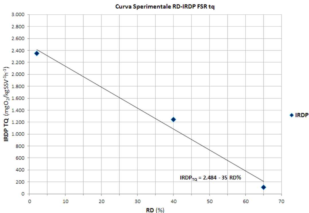
Figura 11. Curva sperimentale correlazione fra tasso di RD e Indice Respirimetrico Dinamico Potenziale (IRDP) del rifiuto tal quale residuale
