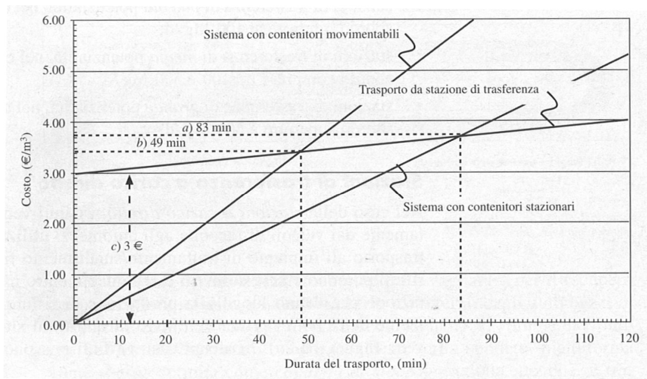
Figura 8 – Esempio di diagramma finalizzato a valutare l'opportunità economica di realizzare una stazione di trasferimento - Manuale "Ingegneria dei Rifiuti Solidi" edito da Hoepli [p.439 – 441]
