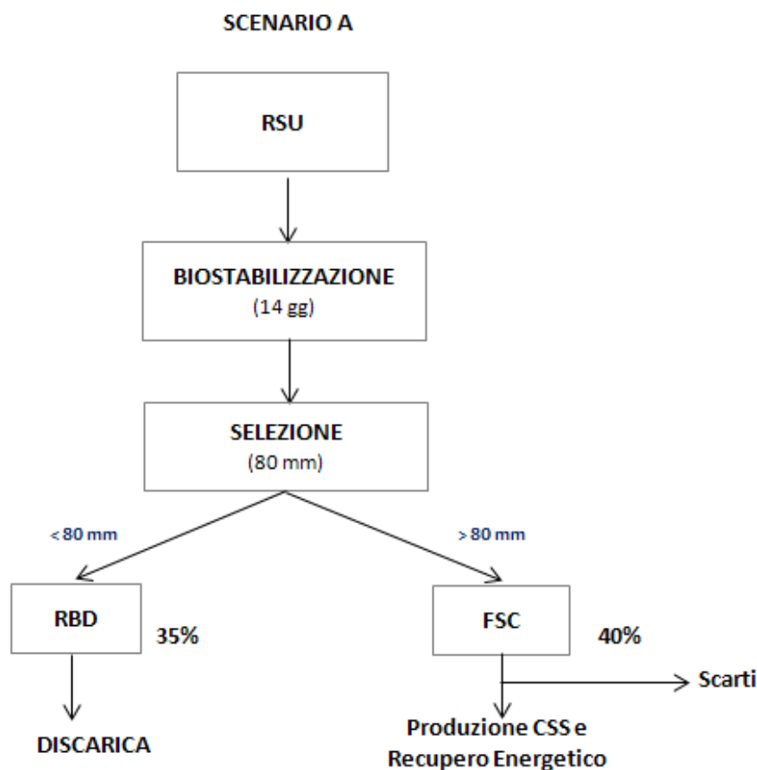
Figura 1. Scenario A. RD \approx 0% e impianto a pieno carico (saturazione potenzialità di trattamento). TMB completo di processo di biostabilizzazione a 14 gg e selezione con produzione RBD e FSC, produzione CSS
